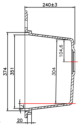
SECTION D-D
